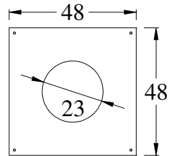
Vue de dessus de la platine (version ouverte)
